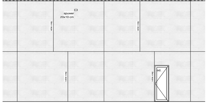
Achtergevel schaal 1:150
